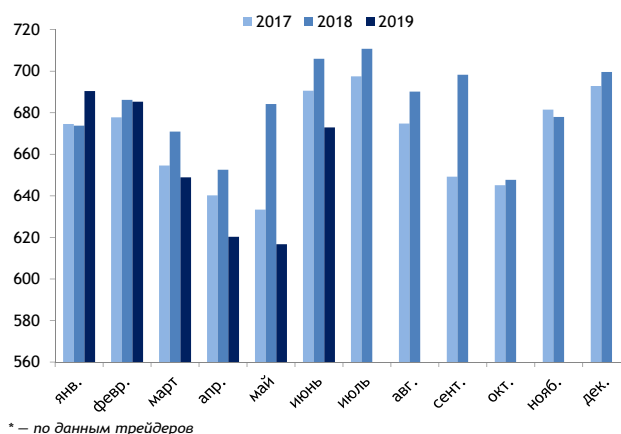
Трубопроводные поставки на НПЗ России тыс. т/сут.
